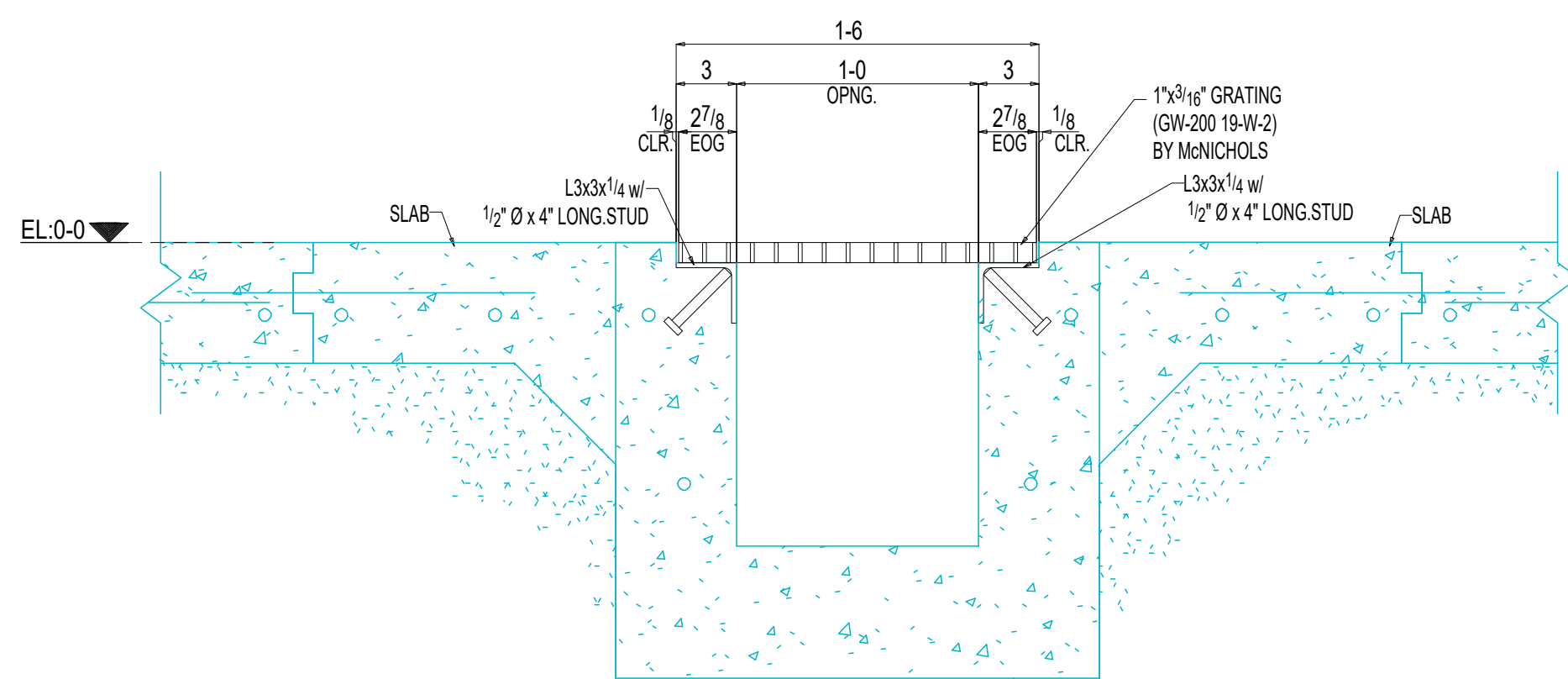
1 SECTION VIEW E13 (REF.DWG. 15/S401)
